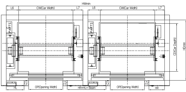
(Passenger / Duplex)
